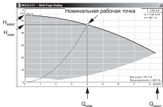
Рис. 93 Показание Q_{ном} , H_{ном} , H_{макс} и Q_{макс}
