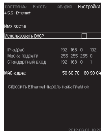
Նկար 130 Ethernet-ի կարգավորման օրինակ
