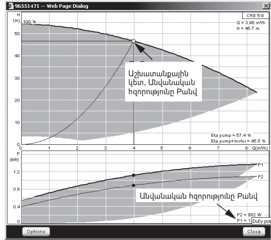
Նկար 96 Անվանական հզորության ցուցումը P անվանական Q անվանական և H անվանական - պոմպերի անվանական աշխատանքային կետ և, որպես օրինք, դա ամենաբարձր ՕԳԳ-ով կետն է:
